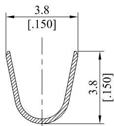
A-A
